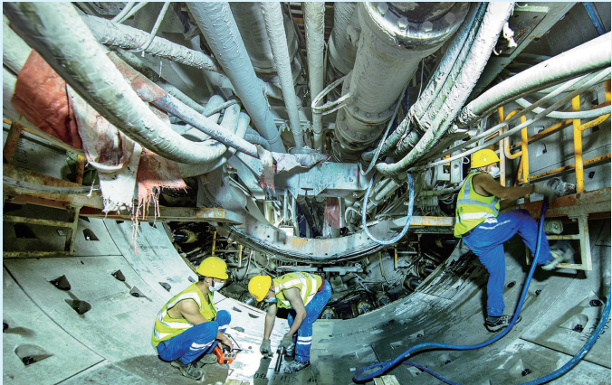
工人在地铁5号线荆农区间施工
